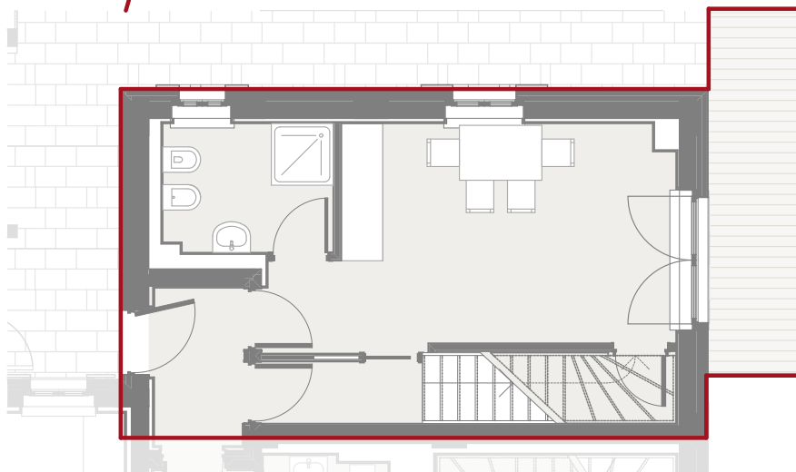
pianta del piano terra
